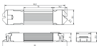
Abmessungen PI-LED LMU
