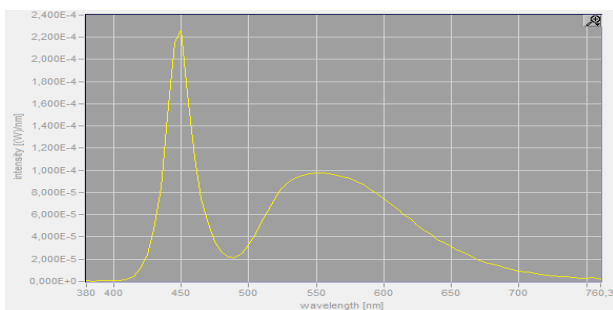
12 Vdc Flex 60 kaltweiß
