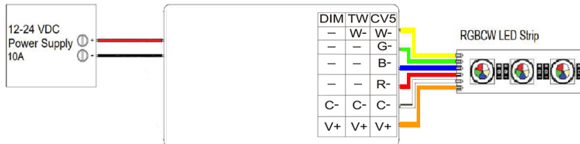
Typisches Schaltbild Typical connection scheme
