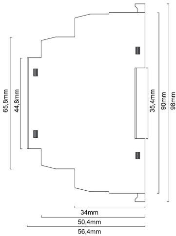
Geometrie 16A Hutschiene
