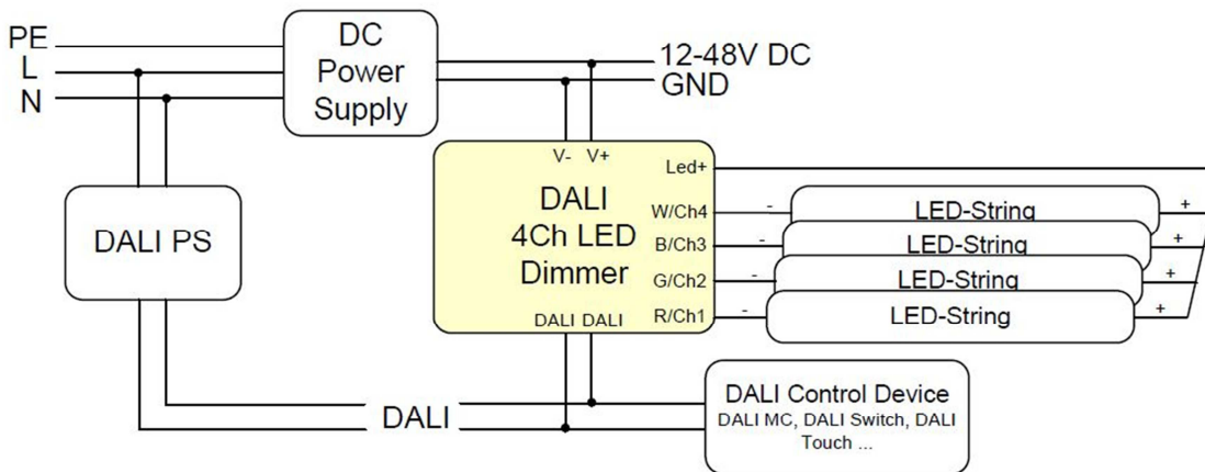
Prinzipschaltbild
